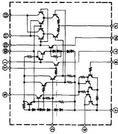
IC201 (LA3301)
