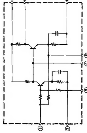
IC101
